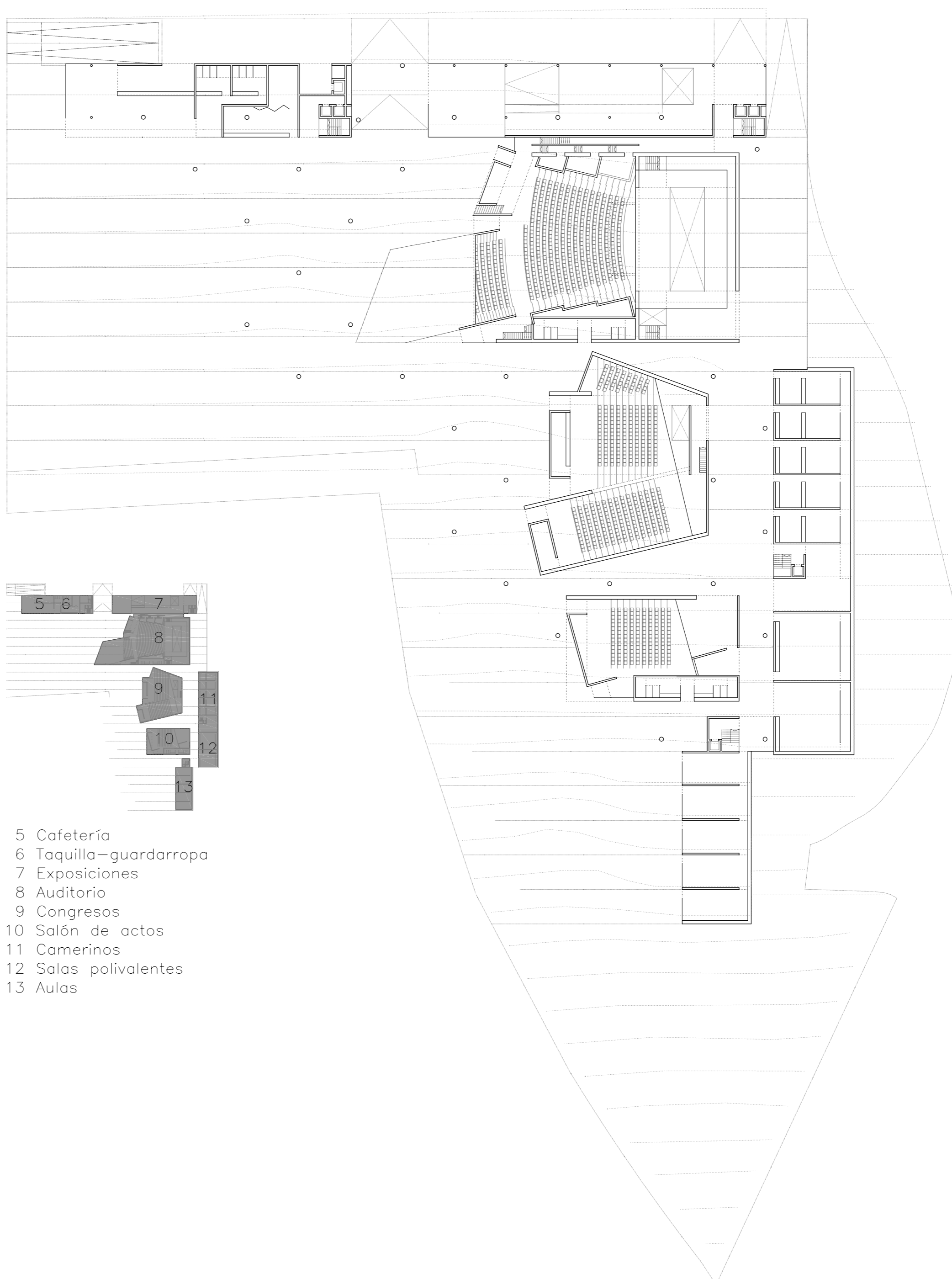
PLANTA BAJA
